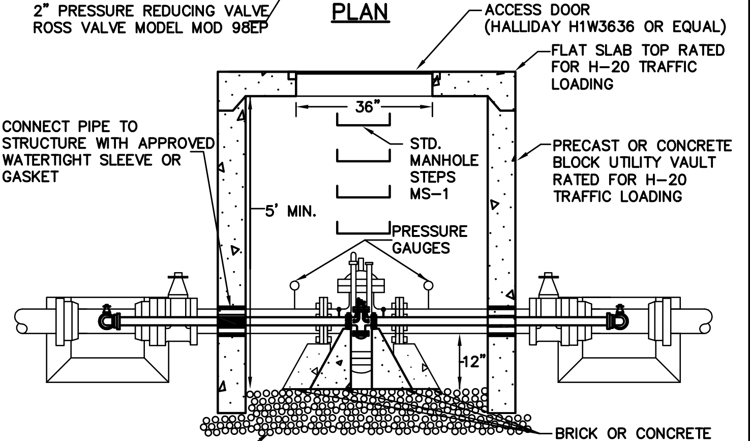
SECTION A-A
